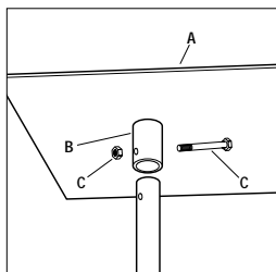
- Detalle 1 - Ensamble la superficie para escritura al poste
