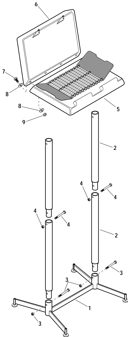
- Detalle 1 - Ensamble el panel para exhibición de catálogos al poste.
