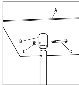
- Detalle 1 - Ensamble el panel para exhibición de catálogos al poste.
